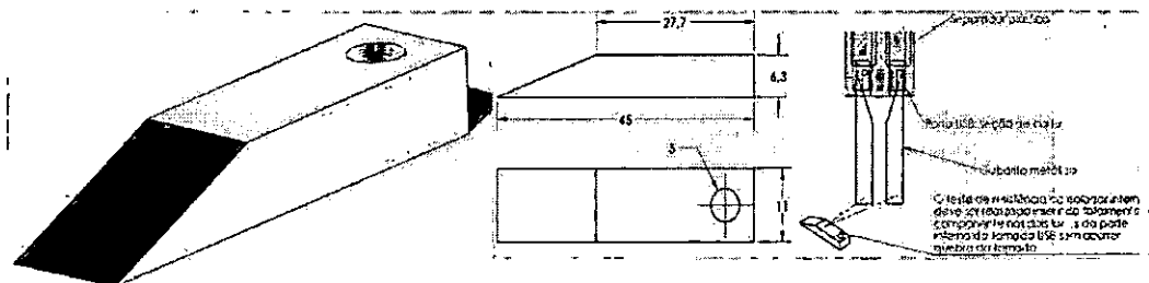
Gabarito para teste de inversão na porta USB Figura 28 – Imagem ilustrativa.
