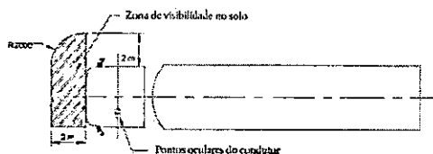
Campo de Visão nº 6 (CV 6)
